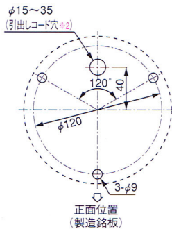
取付寸法 Mounting Dimensions
