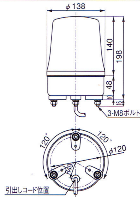
外観寸法図 Dimension
