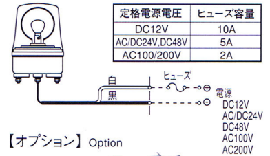
結線図 Wiring
